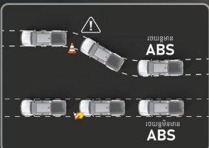
ABS ប្រព័ន្ធជំនួយប្រាំងក្នុងករណី ឈប់បន្ទាន់មិនឲ្យកង់អ្នល និងមិន ចាក់សោរចង្កូត
